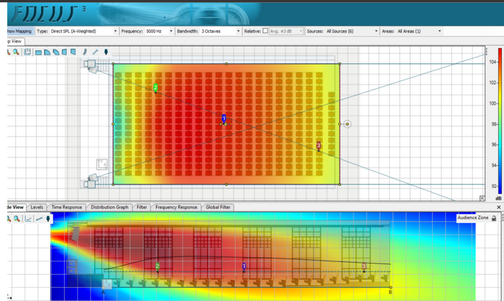
Kierunkowość i rozkład ciśnienia akustycznego w pomieszczeniu
